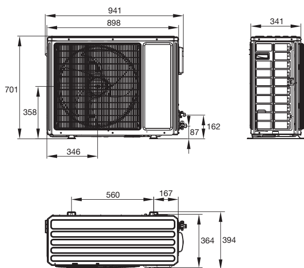
■ GRS-CQ4.0Pd/NhH-E(I) - GRS-CQ10Pd/NhH-E(I)
