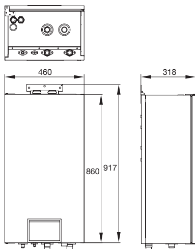
■ GRS-CQ4.0Pd/NhH-E(I) - GRS-CQ10Pd/NhH-E(I)
