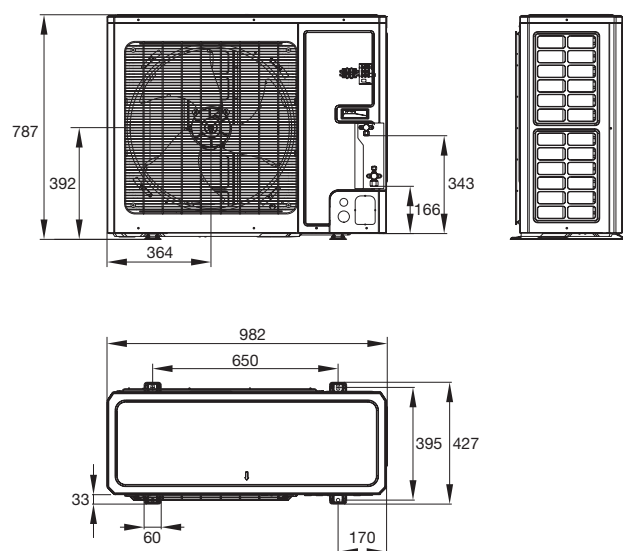
■ GRS-CQ8.0Pd/NhH-E(O) - GRS-CQ10Pd/NhH-E(O)
